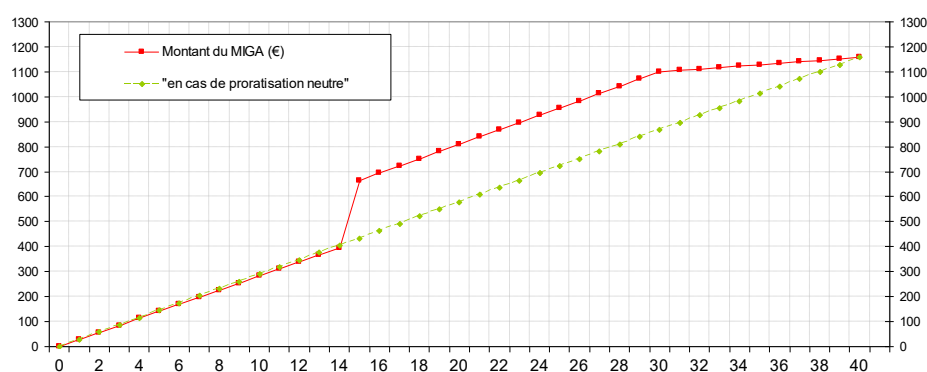
Figure 48 : Proratisation du minimum garanti en fonction de la durée de services effectifs – axe des ordonnées (montant en euros par mois, à partir du 1 er avril 2013 – axe des abscisses)
